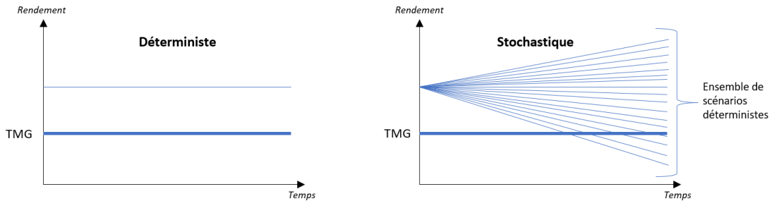
FIGURE 1.7 – Approche déterministe VS approche stochastique
